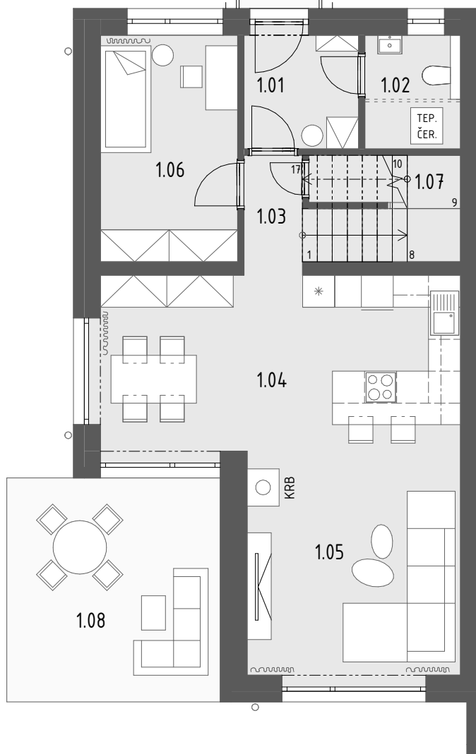
PÔDORYS 1.NP 1 : 100
