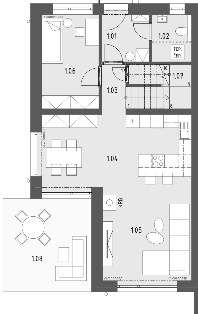
PÔDORYS 1.NP 1 : 100
