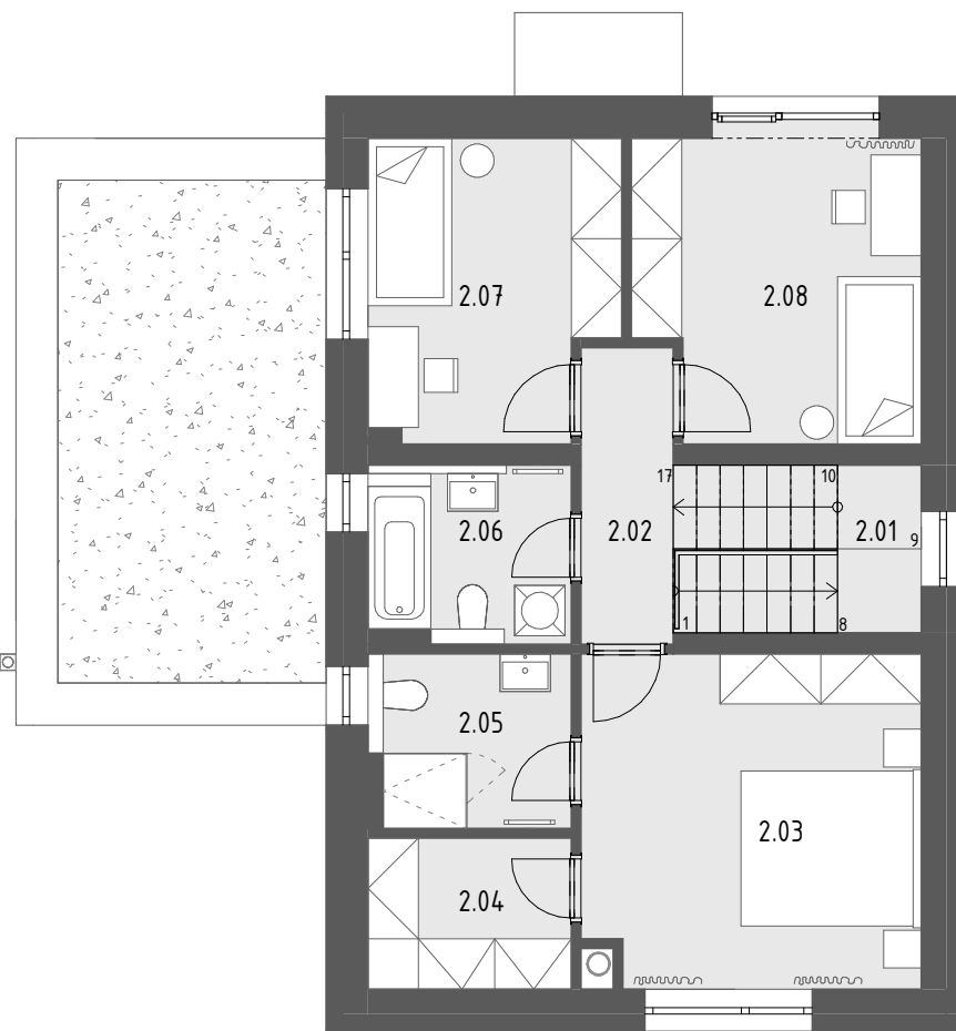
PÔDORYS 2.NP 1 : 100
