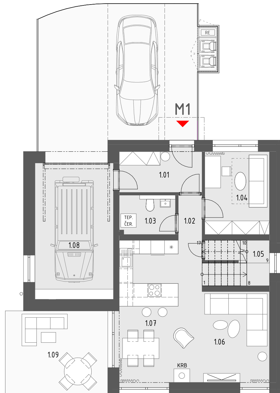
PÔDORYS 1.NP 1 : 100
