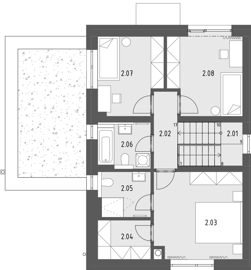
PÔDORYS 2.NP 1 : 100
