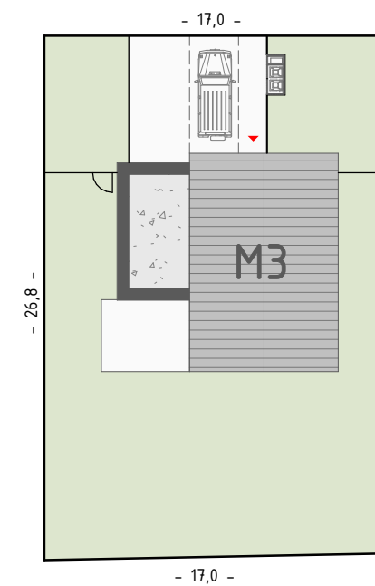
SITUÁCIA 1 : 350
