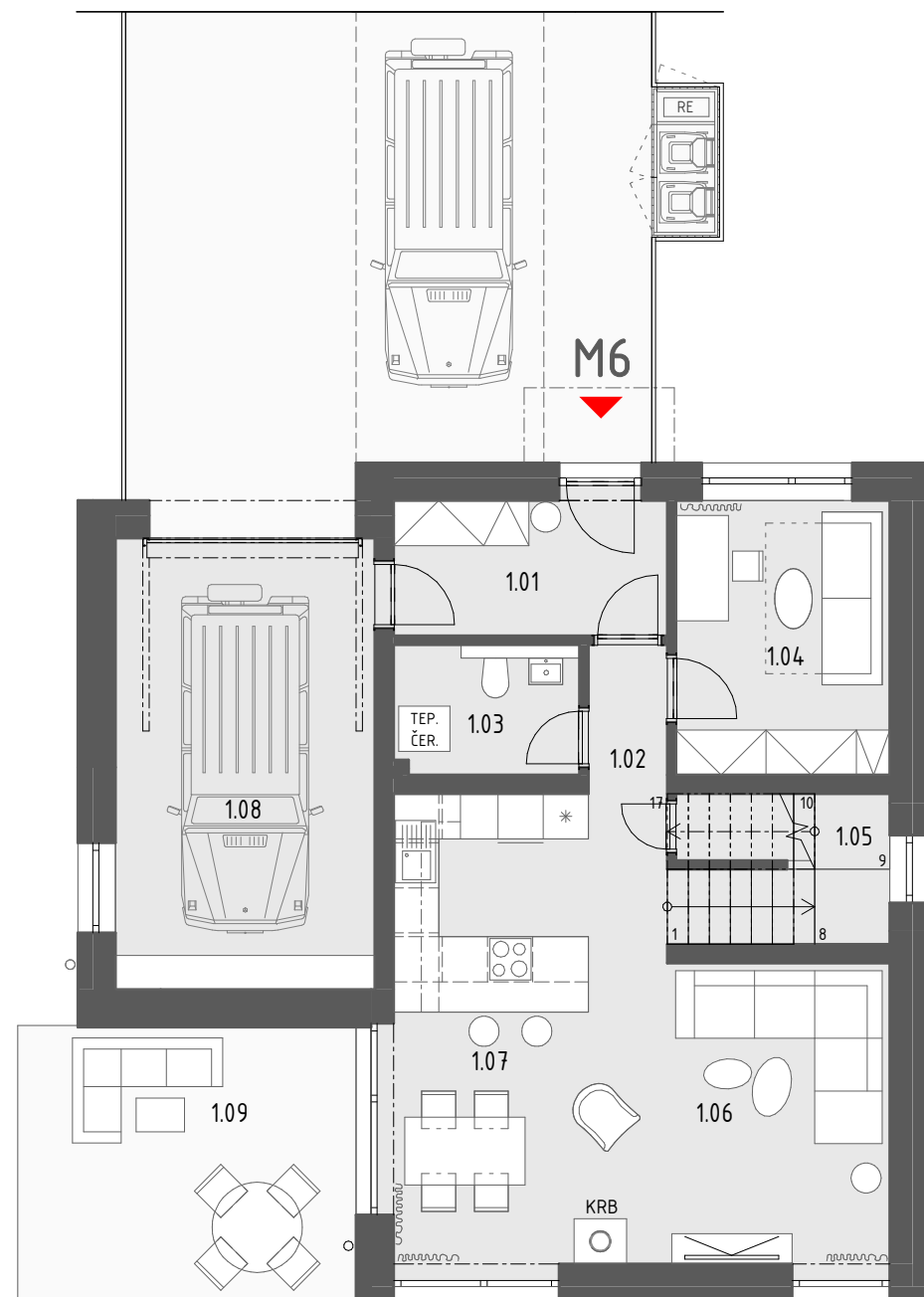
PÔDORYS 1.NP 1 : 100
