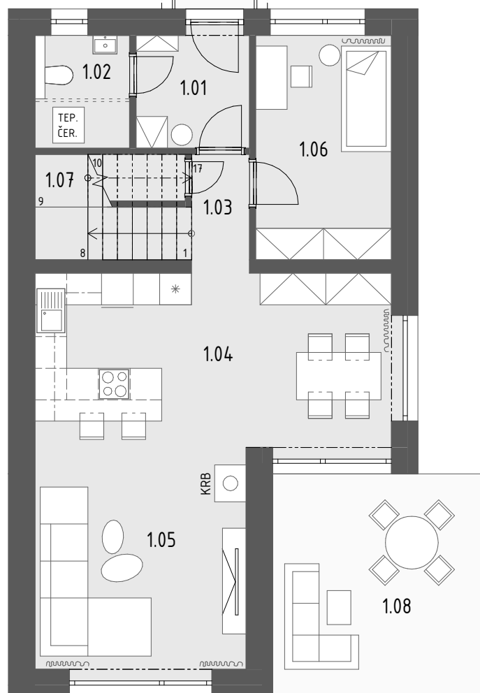
PÔDORYS 1.NP 1 : 100
