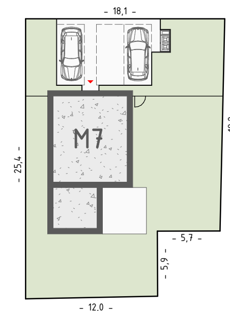
SITUÁCIA 1 : 350
